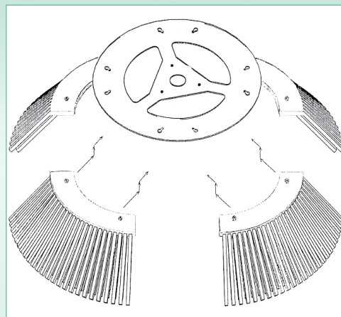
Nastavitelná horní část kartáče, která umožňuje rychlou montáž kartáčů v segmentech
